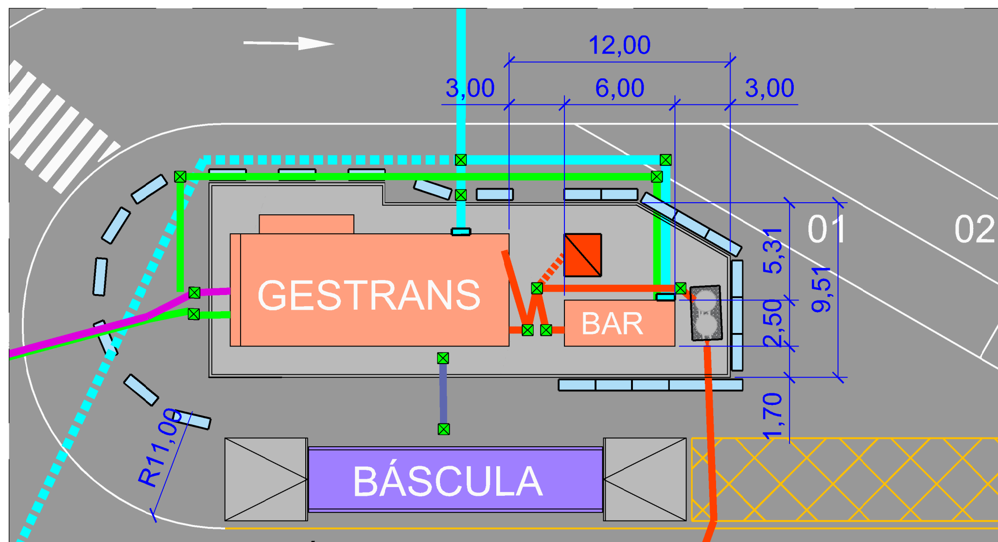
DETALLE A A1_1:200
