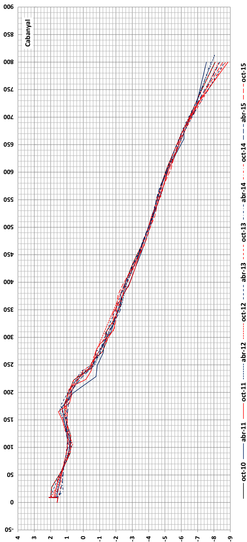
Plan de vigilancia de la evolución de las playas al norte y sur del Puerto de Valencia tras la ejecución de las obras del mismo. Informe 2015.03Final. ANEXO IV. EVOLUCIÓN PLAYA NORTE
